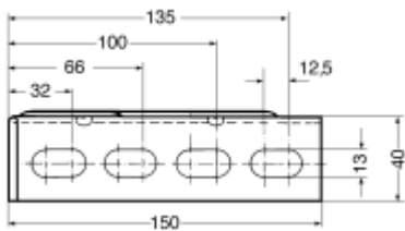
Mensola a squadra WK 150/150
